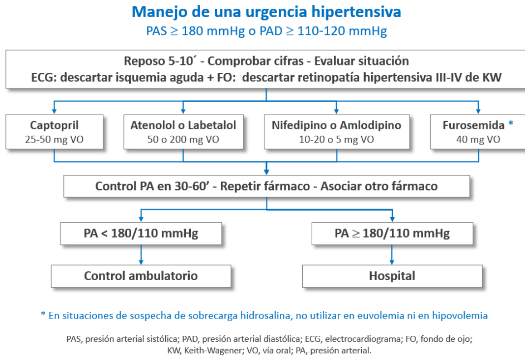
Figura 1. Algoritmo de actuación ante una urgencia hipertensiva
