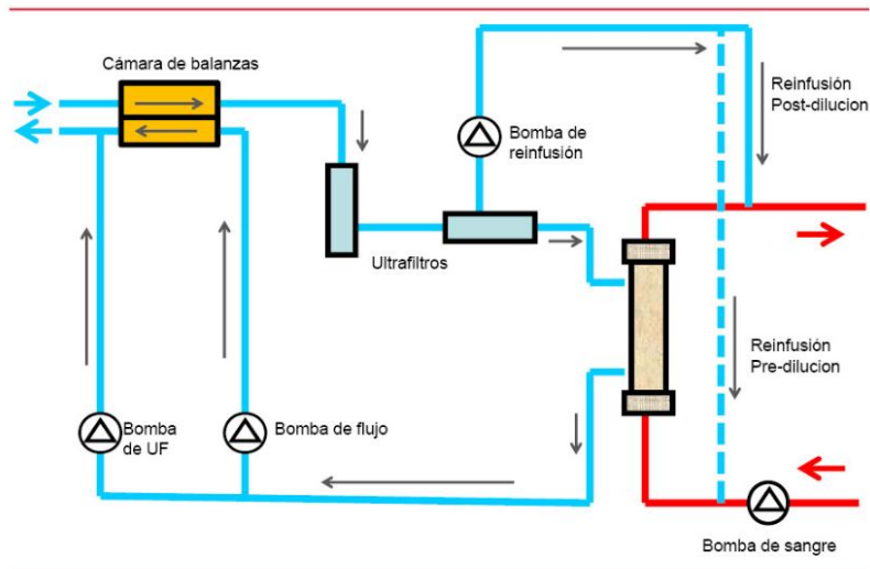
Figura 1. Esquema de funcionamiento de la HDF en línea, en pre y en post dilución
